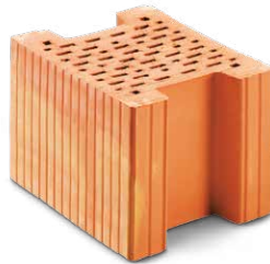
Art. Nr. 262-20 SSZ 25 MT HAG 20
