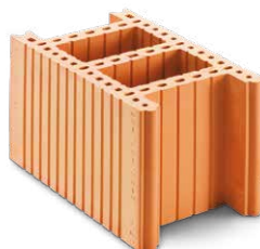
Art. Nr. 565 SSZ Plan-Verfüllziegel 25 HAG 19,9
