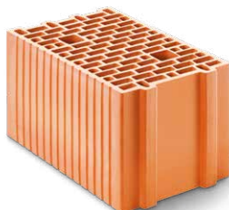
Art. Nr. 524 25 Plan Schwer HAG 19,9
